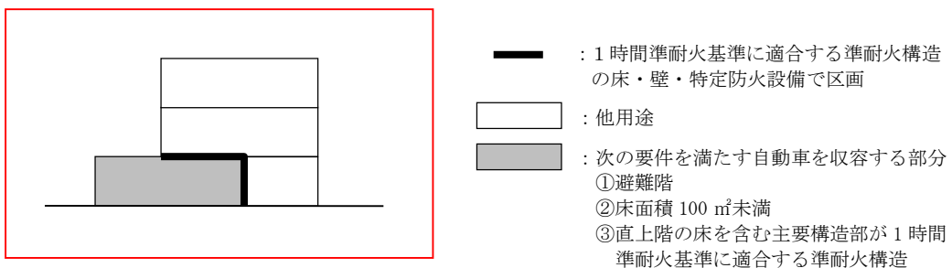
図 52-5 第2号の規定の区画例
