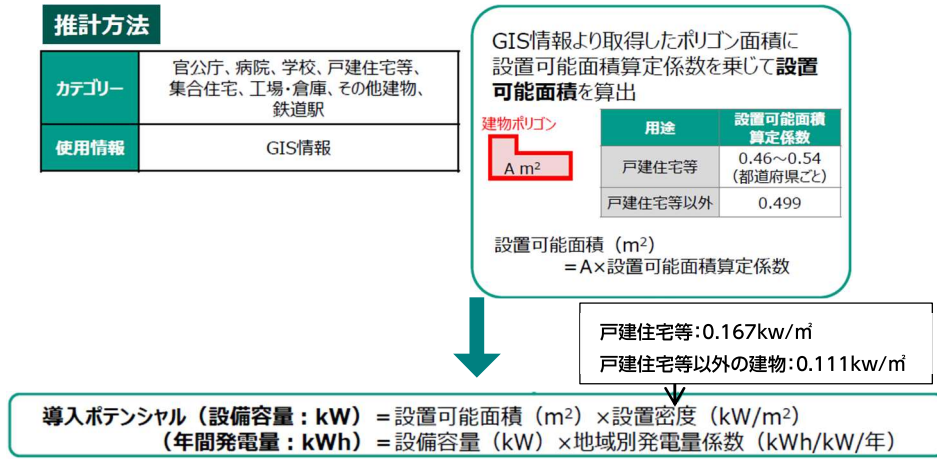
図 2-4 REPOS による太陽光の導入ポテンシャルの算定方法
